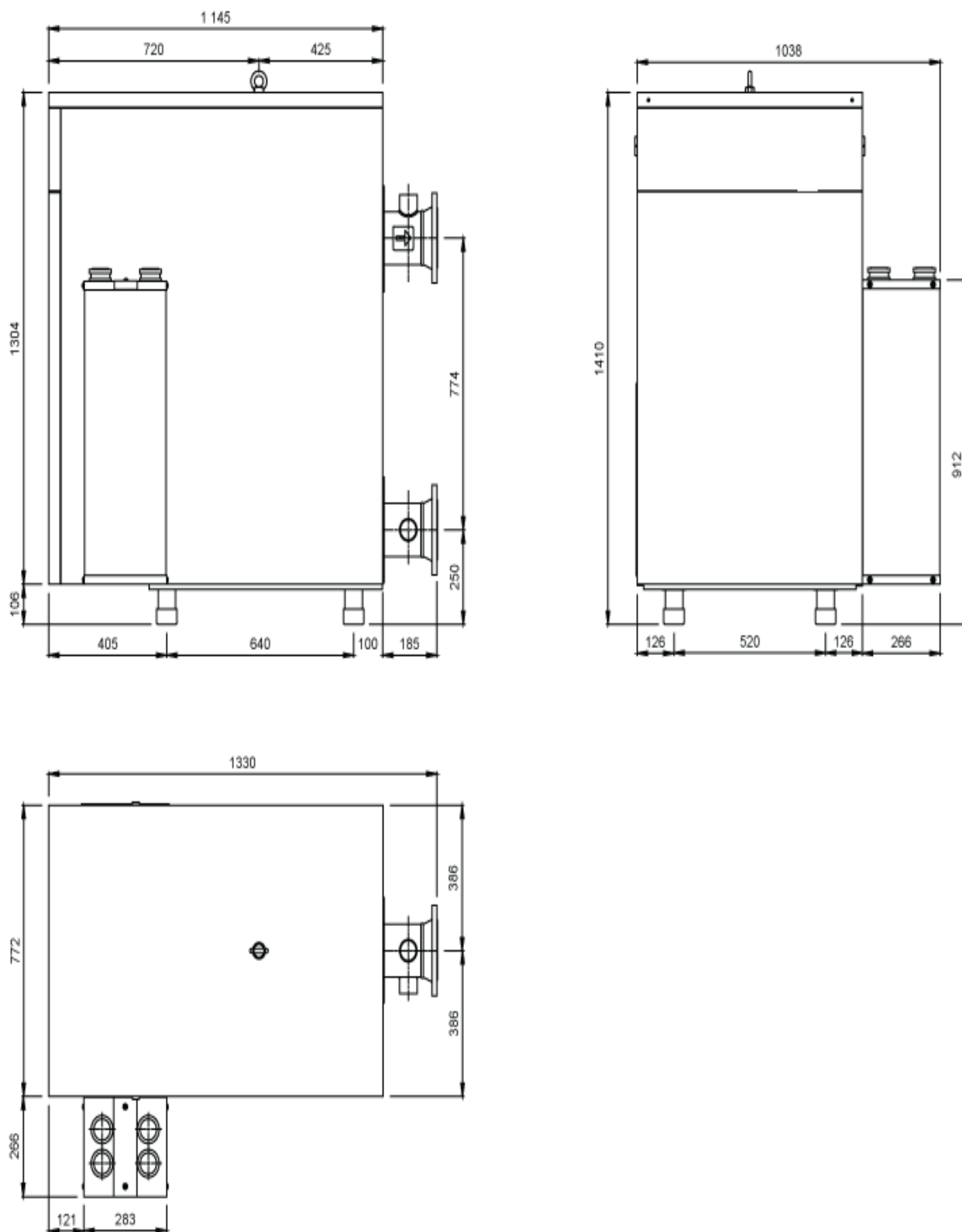
Fig. 1 Schița și dimensiunile cazanului condiționate de locul de montaj și instalația existentă:
